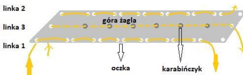
Rysunek 2. Proponowany sposób montażu żagla (trzecia linka jest opcjonalna).
