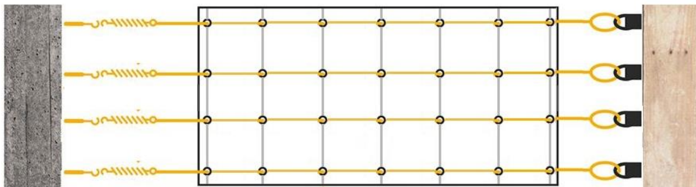
Rys 1. Poprawne mocowanie rolety poziomej
